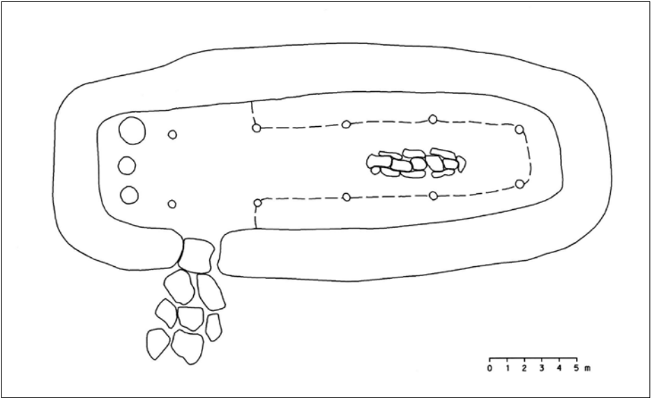
Hugsanlegt útlit víkingaaldarskála á Öndverðareyri.
