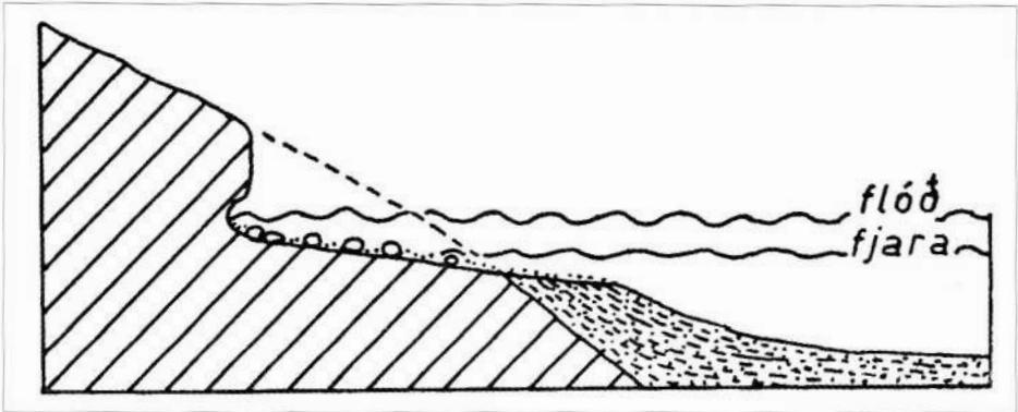
Brimstallar. Stríklínan sýnir upphaflega hlíð. Lóðrétti veggurinn nefnist brimklif, en lárétti pallurinn brimþrep. Fyrir framan það myndar bergmylsnan skálögóttan marbakka.
