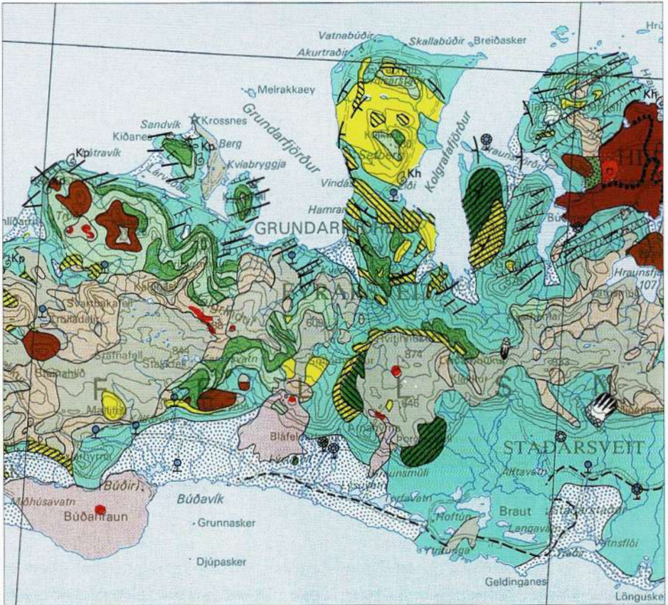
Hluti af jarðfræðikorti af Íslandi, blaði 2, Mið-Vesturland. Haukur Jóhannesson, 1994, Náttúrufræðistofnun Íslands og Landmælingar Íslands.
